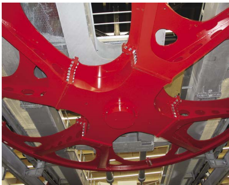
Die Doppelmayr-Entwickler schufen völlig neuartige Konstruktionen für die Seilscheibe und die Rollenbatterie zum Transport der vom Seil abgekuppelten Kabinen und reduzierten so Lärm und Vibration auf vernachlässigbare Werte.
